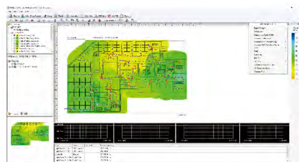
802.11 熱圖
